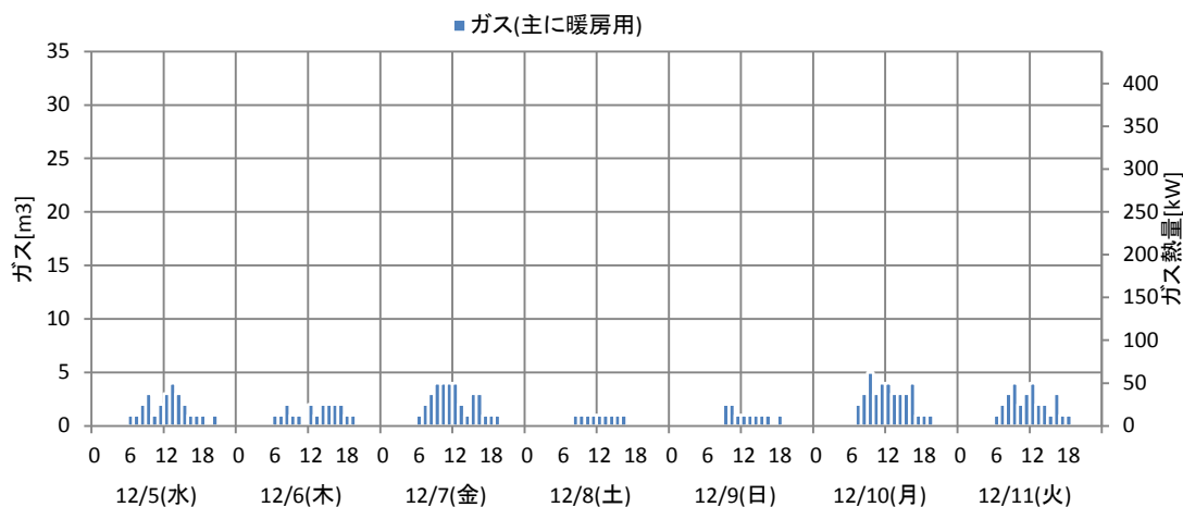
図 4-11 ガスの変動
