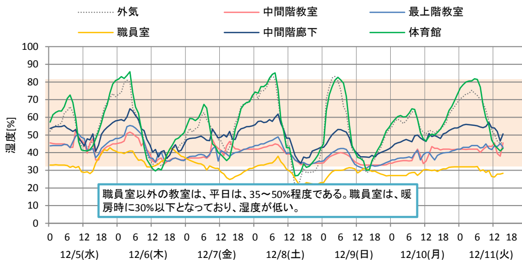
図 4-14 湿度変動
