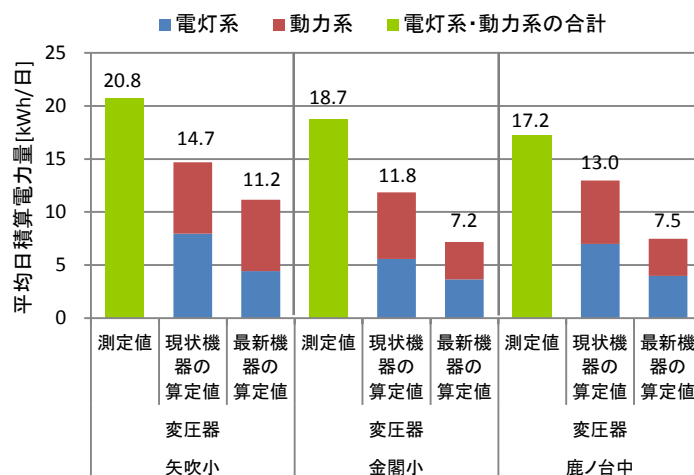
図 5-18 変圧器の日積算電力量(損失)の比較
