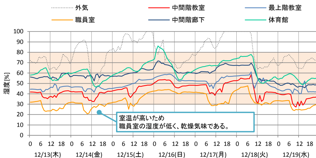
図 2-12 湿度変動
