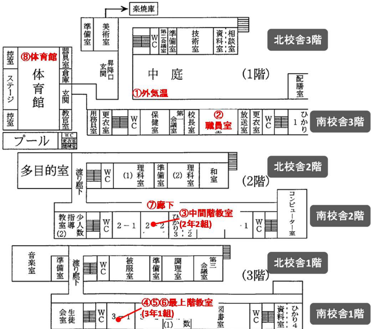
図 4-6 測定ポイント
