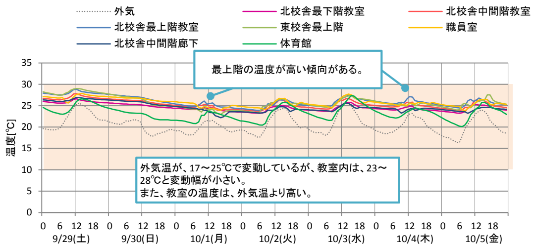
図 3-10 温度変動
