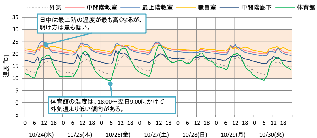
図 4-9 温度変動
