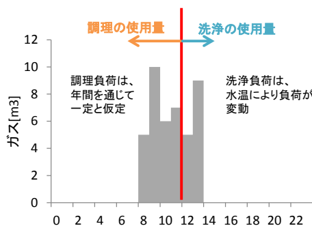
調理と洗浄によるガス消費量(暖冷房の使用がない日)の変動
