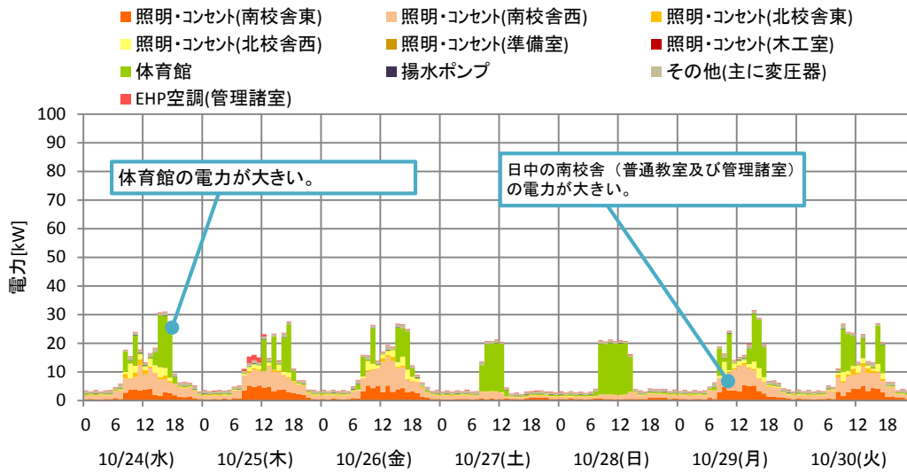
図 4-7 電力の変動
