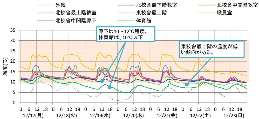
図 3-13 温度変動
