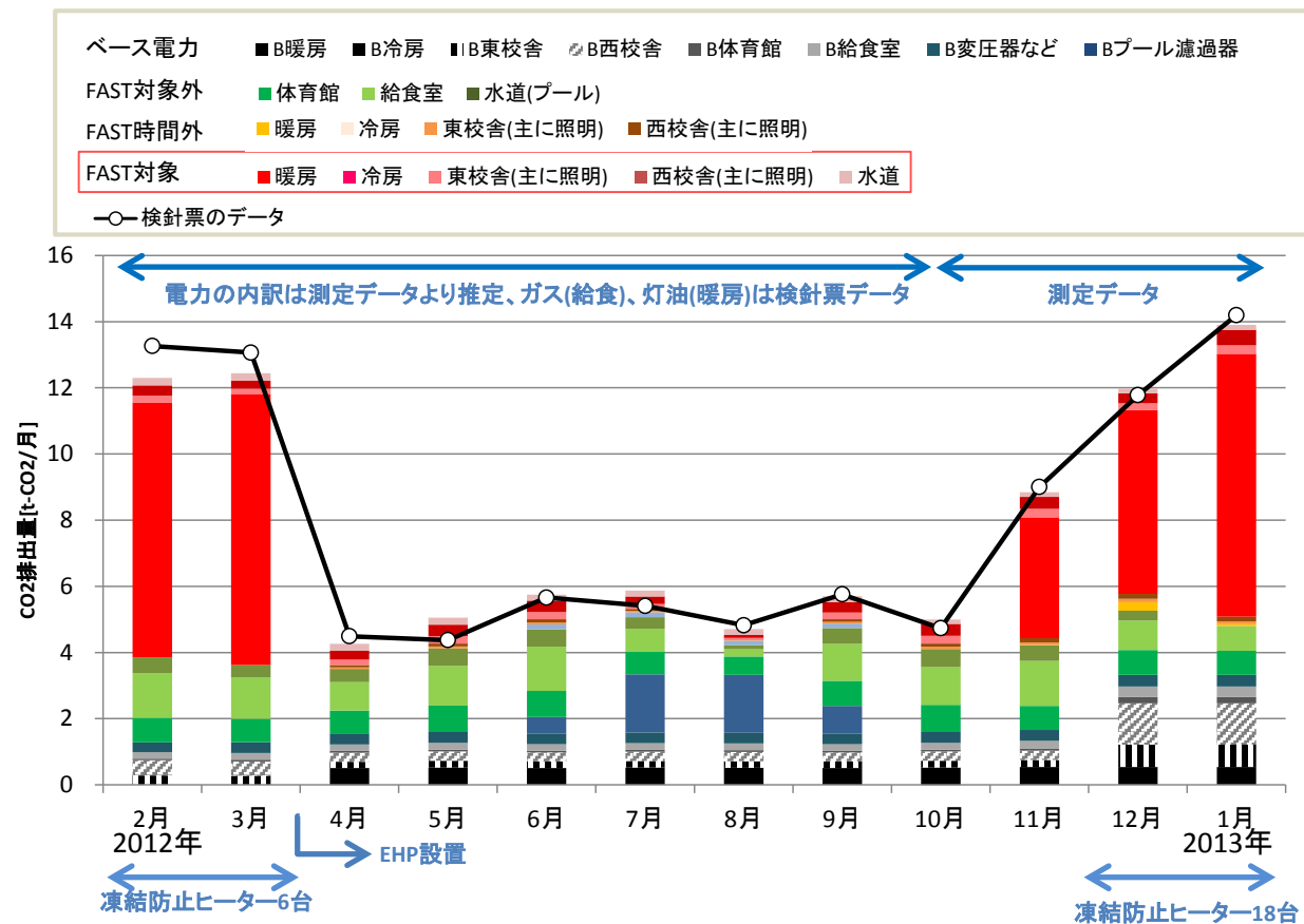
図 2-41 月別 CO2 排出量の内訳推定結果
