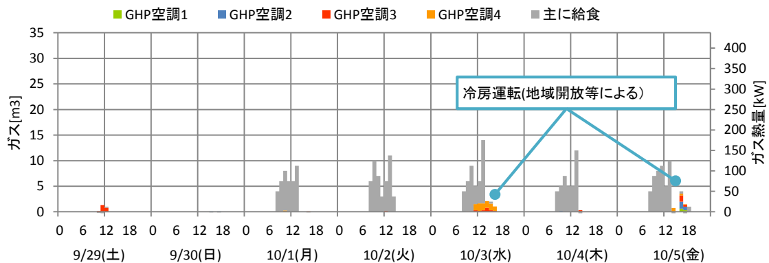
図 3-9 ガスの変動
