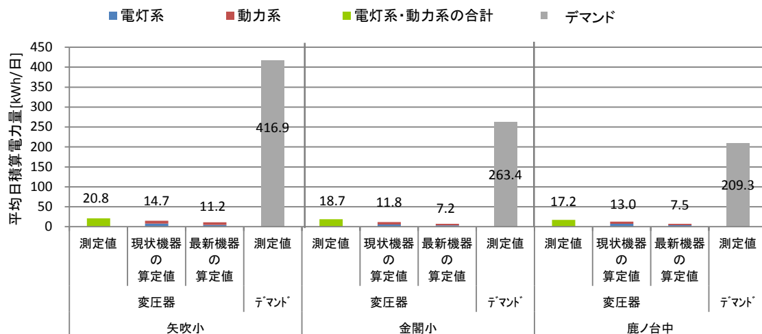
図 5-19 デマンドに対する変圧器の割合
