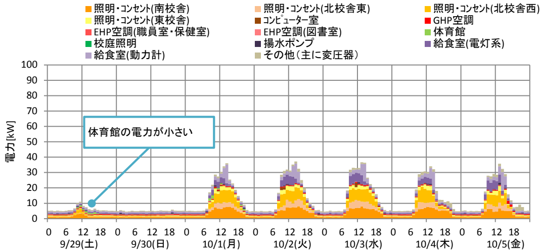
図 3-8 電力の変動
