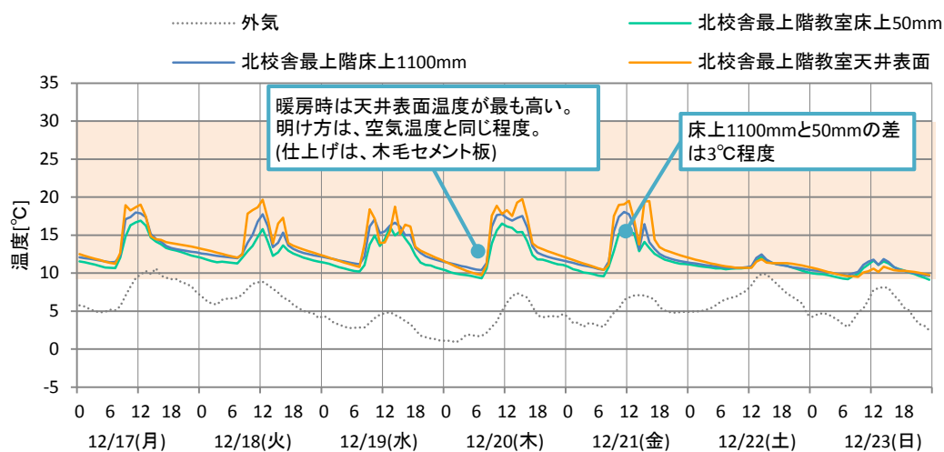
図 3-15 最上階教室の温度変動
