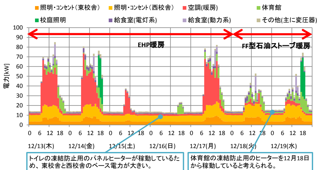
図 2-9 電力の変動
