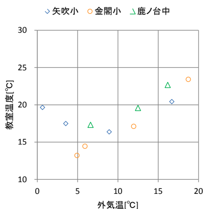
図 5-32 月平均外気温と月平均教室温度の関係
